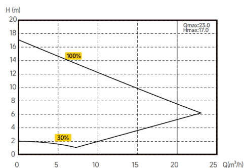
ydelseskurve
